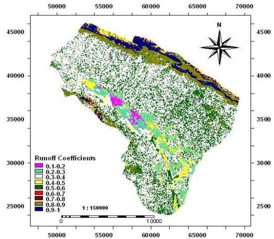
شکل شماره ۵: نقشه ضریب رواناب سال ۱۳۵۴
