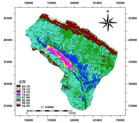
شکل شماره ۳: نقشه شماره منحنی سال ۱۳۶۹
