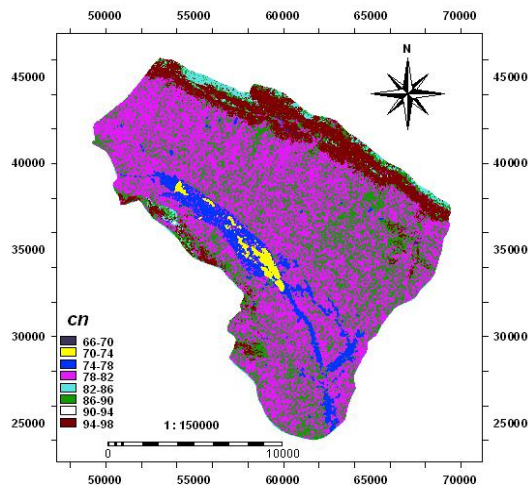
شکل شماره ۴: نقشه شماره منحنی سال ۱۳۸۵
