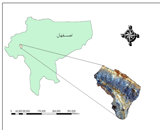
شکل شماره ۱: موقعیت منطقه مطالعاتی در استان اصفهان
