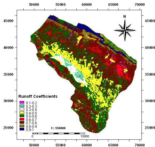
شکل شماره ۷: نقشه ضریب رواناب سال ۱۳۸
