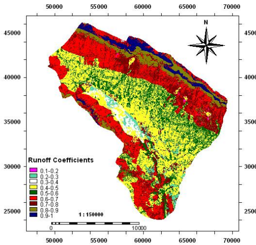
شکل شماره ۶: نقشه ضریب رواناب سال ۱۳۶۹
