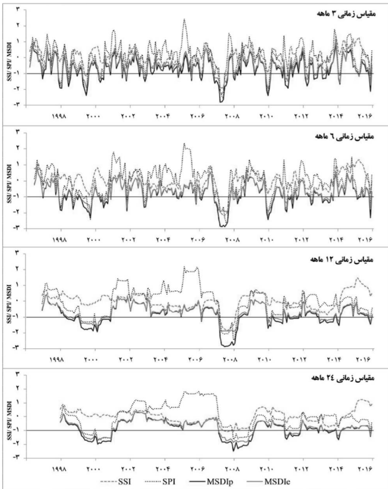
شکل ۴. مقادیر شاخص‌های SSI، SPI، MSDIp، MSDIe در استان چهارمحال و بختیاری از ۱۹۹۷ تا ۲۰۱۶ (رنگی در نسخه الکترونیکی)
